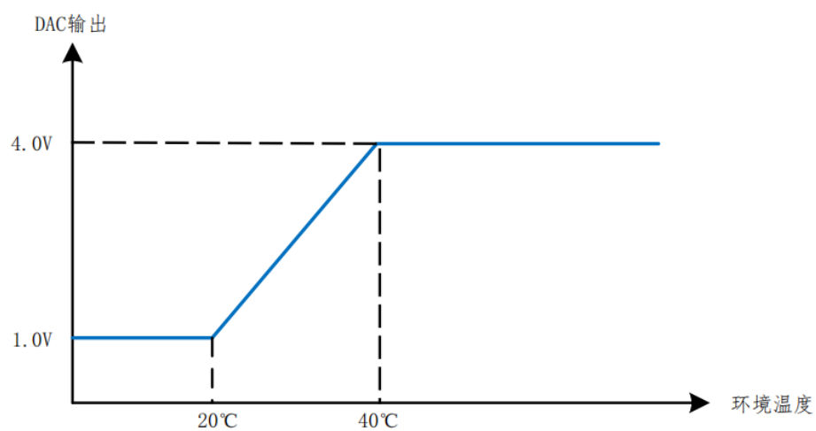
图 7 模式 2 下 DAC 输出电压
